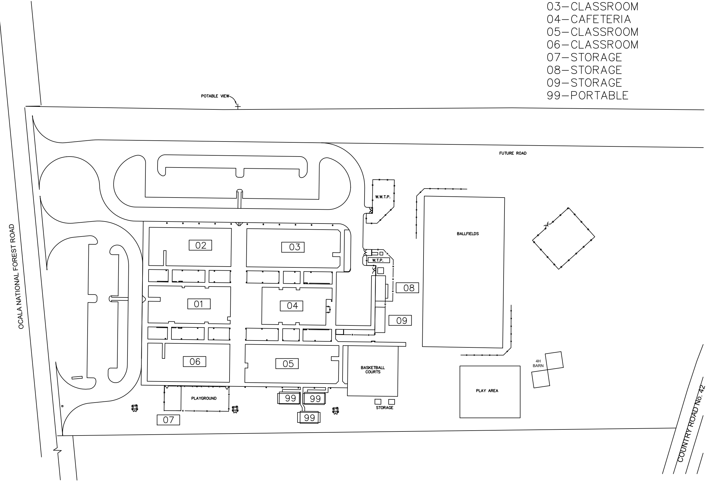
1 OVERALL SITE PLAN SP-02 SCALE: N.T.S.
